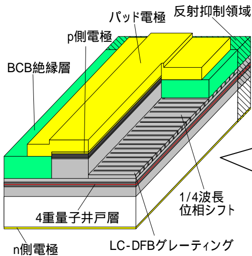
レーザ構成図
