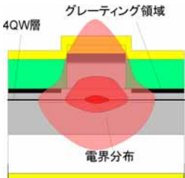
レーザ構成図
