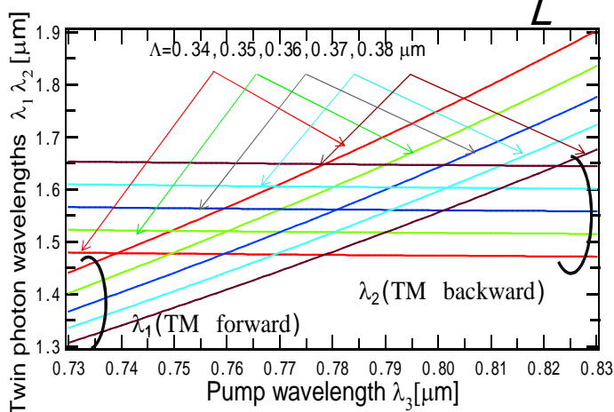
ポンプ光波長と光子対波長の関係 (TYPE 1次QPM)
