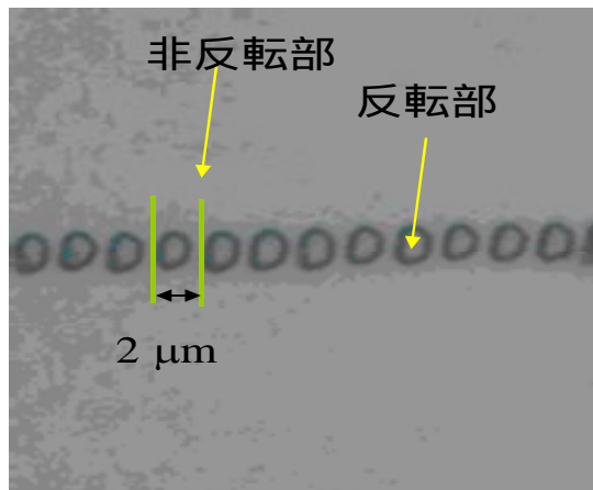
周期分極反転構造(電極端部分)
