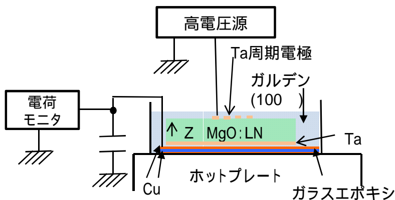
電圧印加セットアップ
