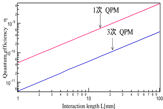
相互作用長と量子効率の関係
